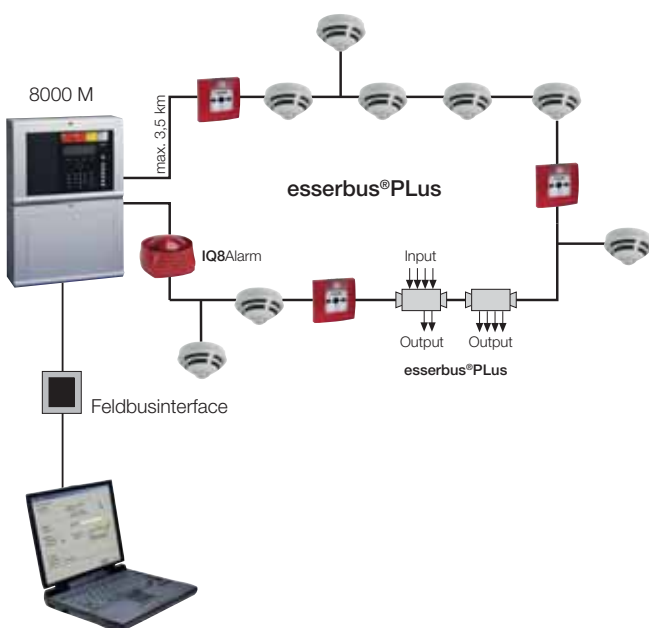
Funktionstest über BMZ
